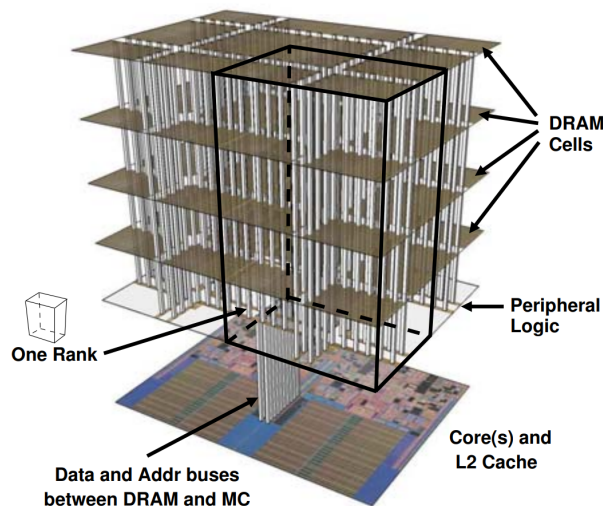
FIGURE 1.11 – Intégration d'une architecture multicœur 2D au sein d'une architecture multiplans 3D. Les Through-Silicon Vias (TSVs) permettent de connecter les plans entre eux à de multiples endroits pour obtenir une large bande passante[Loh08].
