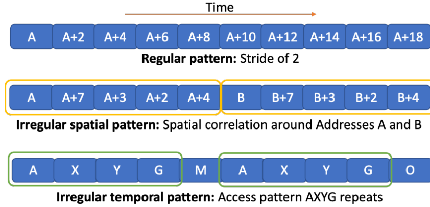
FIGURE 1.7 – Motifs d'accès à la mémoire détectés par différents types de mécanismes de prefetching. Image tirée de [Arm].
