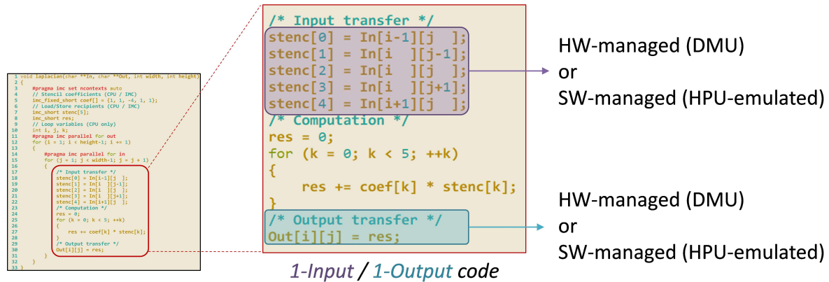
FIGURE 5.10 – Le code de l'opérateur laplacien présenté en exemple possède après analyse un flux d'entrée et un flux de sortie, chacun pouvant être associé à canal de transfert différent.
