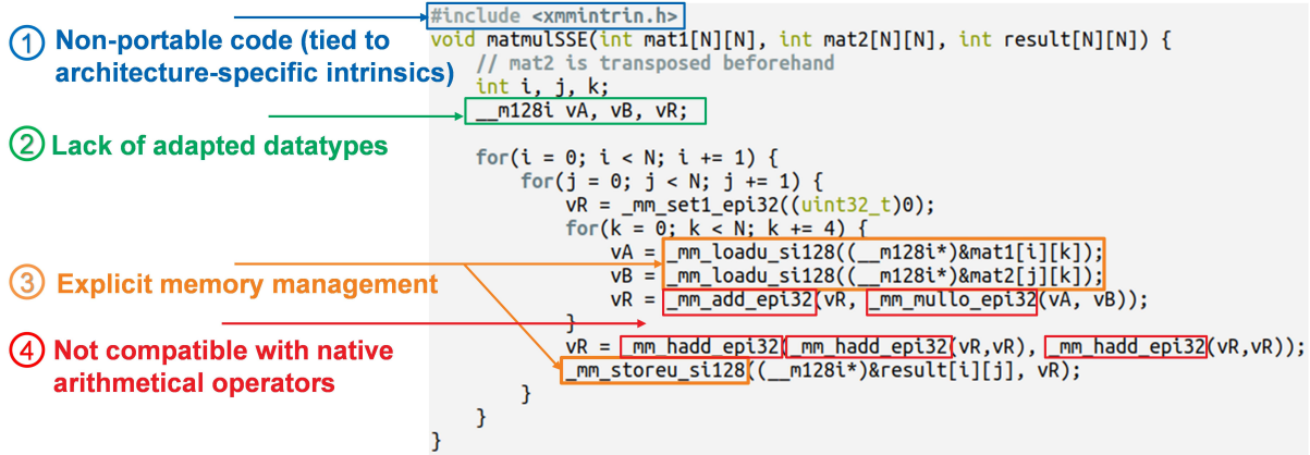
FIGURE 2.2 – L'implémentation de la multiplication matricielle avec l'API xmmintrin.h pour les architectures Intel SSE/AVX. Deux modèles d'exécution sont syntaxiquement présents dans le code (scalaire/SIMD).
