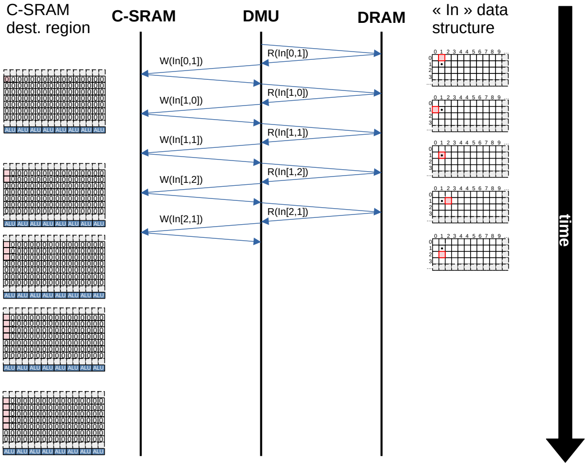
FIGURE 4.5 – Exemple du transfert d’une croix de stencil de la DRAM vers la C-SRAM, avec le DMU.
