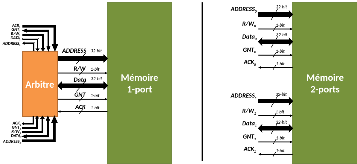
FIGURE 4.7 – L'utilisation de mémoires 2-port permet la réception de requêtes concurrentes de données émises par le DMU et le HPU. Dans le cas contraire un arbitre doit être intégré pour prioriser les requêtes émises par le HPU.
