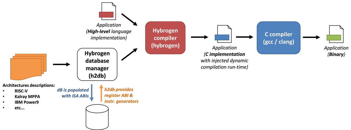
FIGURE 3.10 – Le flot de compilation de Hybrogén permet de programmer des kernels dynamiquement compilés.
