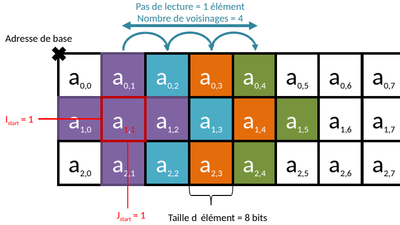
FIGURE 4.2 – Première partie des paramètres du transfert de données présenté lors de la Figure 4.1. Les croix de stencil d'éléments 8 bits sont lues depuis la mémoire DRAM avec un pas de lecture d'un élément.
