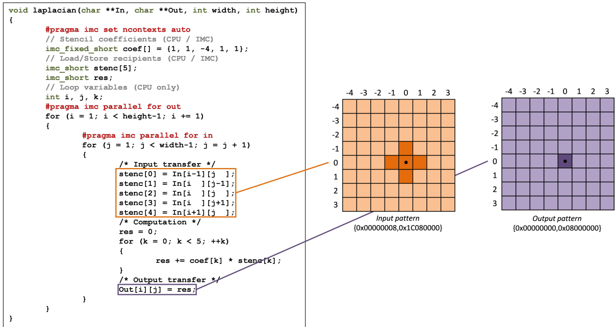
FIGURE 5.4 – Les clauses supportées par le modèle de programmation IMCCC permettent d'exprimer le transfert de données de stencils de façon explicite et pouvant être analysée par un compilateur.
