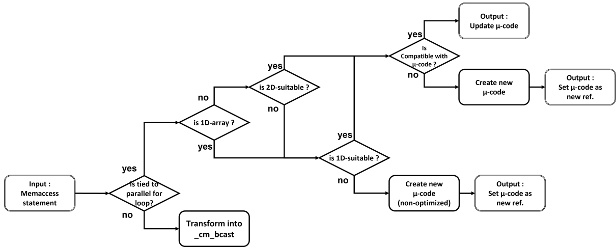
FIGURE 5.8 – Algorithme d'association des clauses d'accès mémoires.
