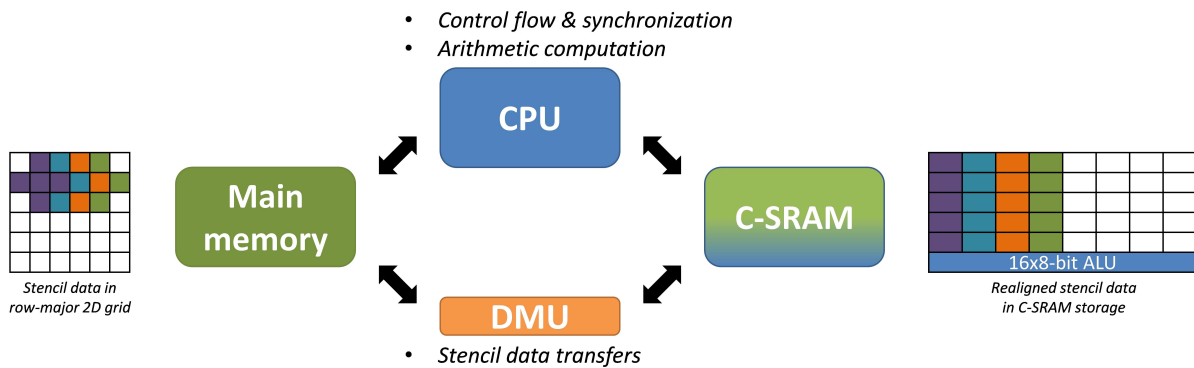
FIGURE 4.1 – L'intégration du Data-locality Management Unit (DMU) permet de décharger le HPU de la tâche de transférer et réorganiser les données de stencils tout en le permettant de paralléliser le transfert de données avec du calcul en C-SRAM.
