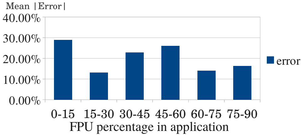
FIGURE 5.3 – Erreur du modèle pour estimer la dégradation. L’erreur est stable par rapport au pourcentage d’utilisation.
