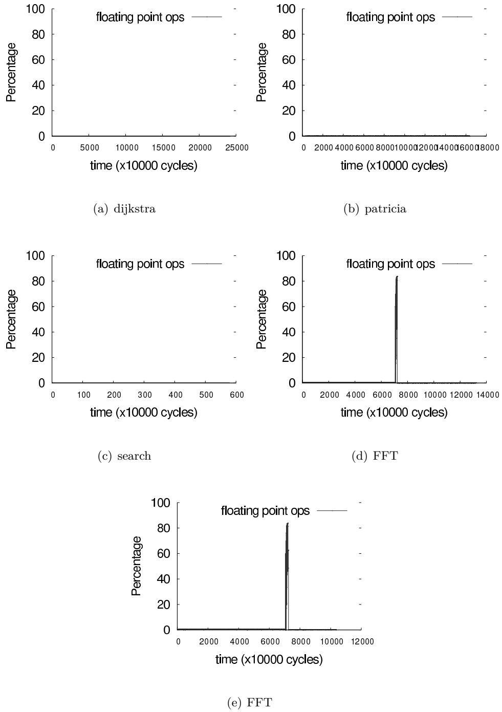
FIGURE C.8 – Profils Mibench - Utilisation de l'unité flottante (FPU) de ARM pendant l'exécution. Chaque point du graphique est une moyenne sur 10K cycles. Il y a des phases de programmes distinctes pour l'utilisation de la FPU .
