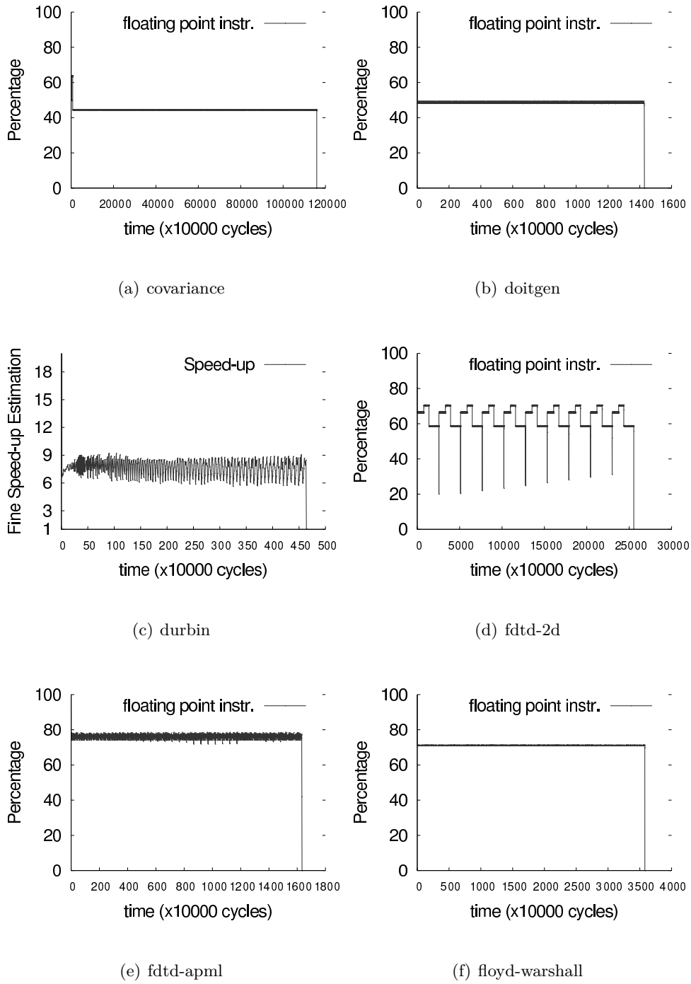
FIGURE C.2 – Profils Polybench - Utilisation de l'unité flottante (FPU) de ARM pendant l'exécution. Chaque point du graphique est une moyenne sur 10K cycles. Il y a des phases de programmes distinctes pour l'utilisation de la FPU.
