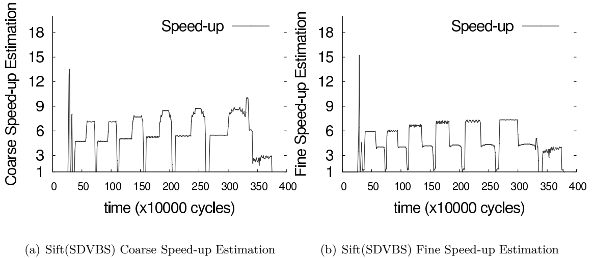
FIGURE 5.4 – Estimation de l'accélération avec la méthode grossière (a) et la méthode fine (b) pour l'application Sift (Chaque point du graphique est l'estimation pour un quantum de 10K cycles).
