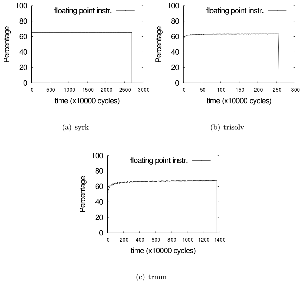
FIGURE C.5 – Profils Polybench - Utilisation de l'unité flottante (FPU) de ARM pendant l'exécution. Chaque point du graphique est une moyenne sur 10K cycles. Il y a des phases de programmes distinctes pour l'utilisation de la FPU .
